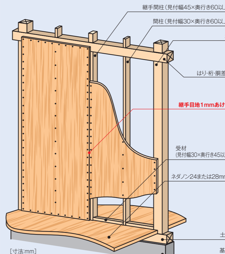
施工例3 合板を高さ方向に張り継がない場合
