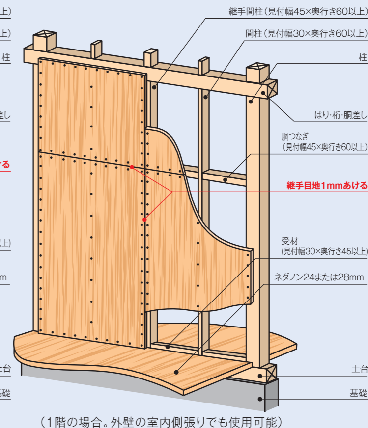
施工例4 合板を高さ方向に張り継ぐ場合
