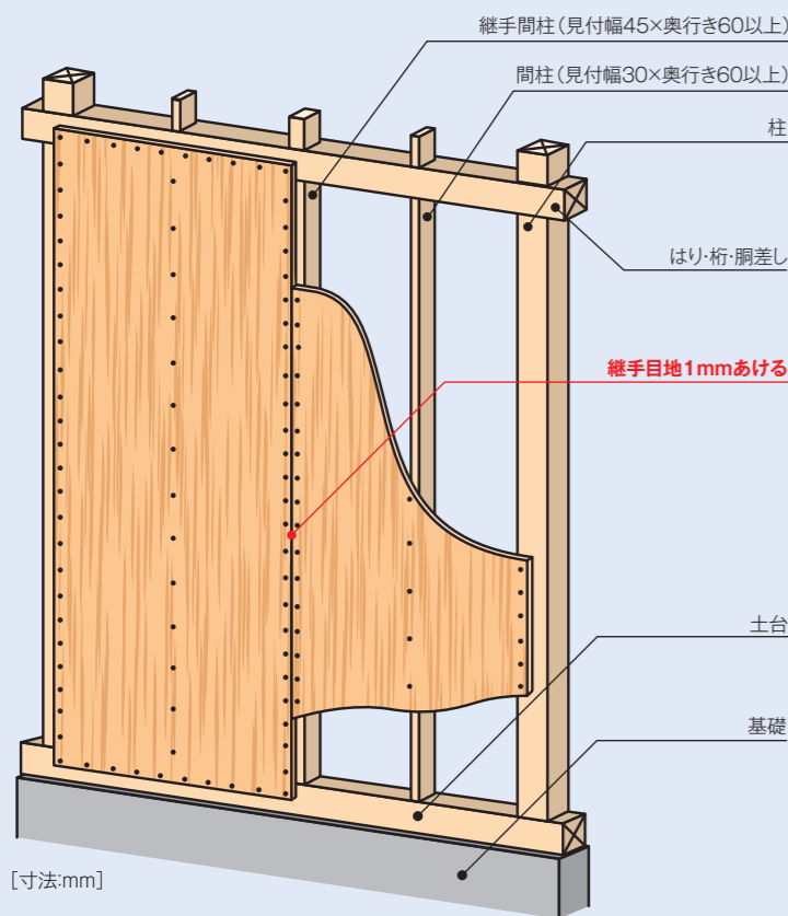
施工例1 合板を高さ方向に張り継がない場合
