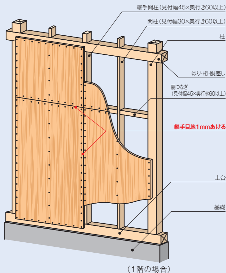
施工例2 合板を高さ方向に張り継ぐ場合
